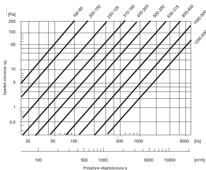
3 stopień redukcji
