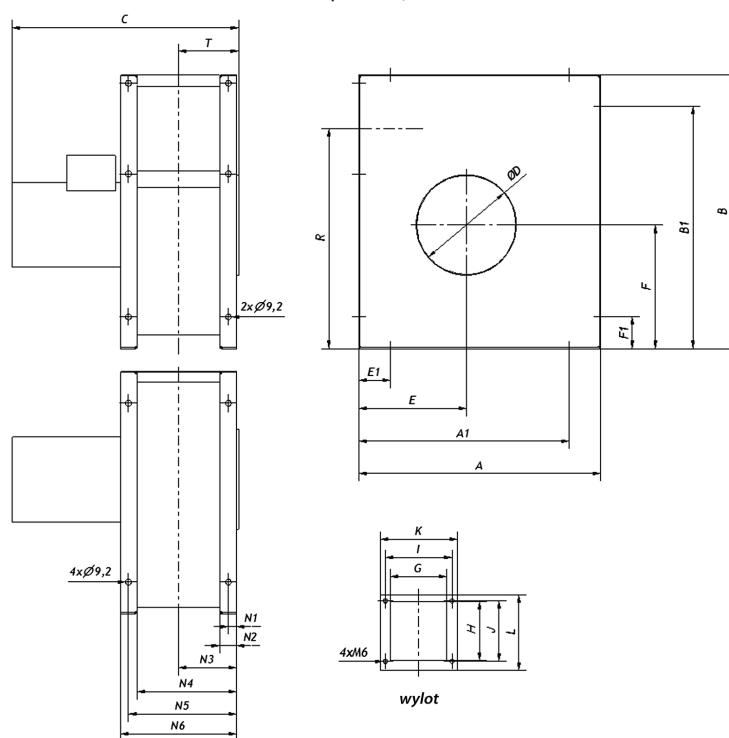
GMT 60-400 obudowa prostokątna
