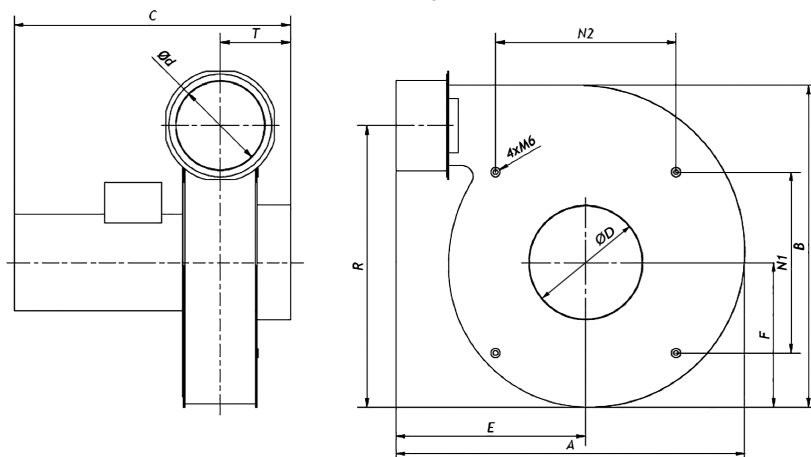
GMT 100-130 obudowa spiralna
