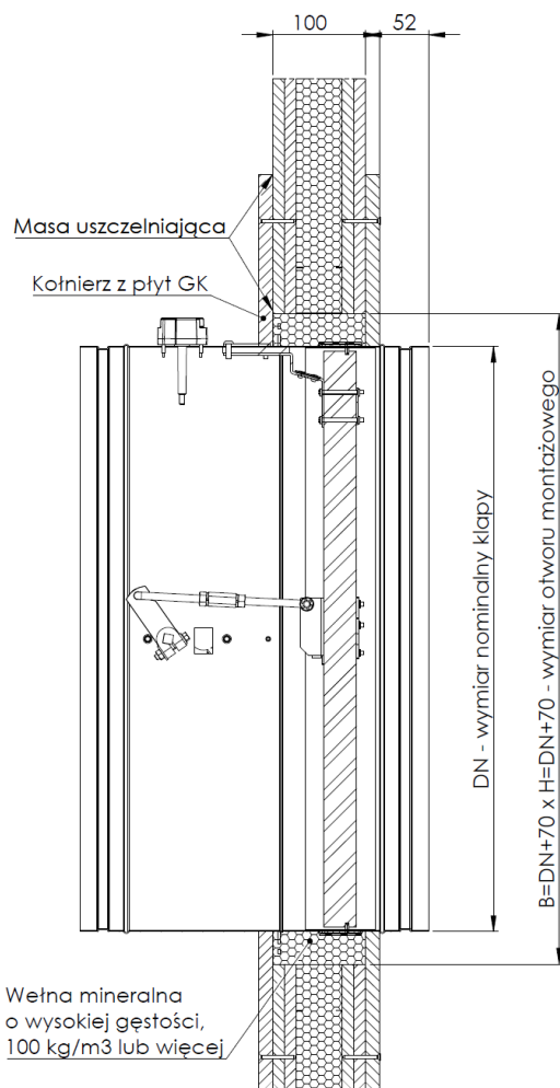
Rys.10. Sposób zabudowy kłap odcinających KTS w podatnych konstrukcjach ściennych o grubości 100 mm
