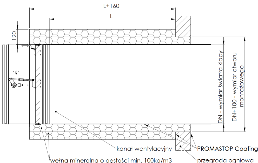
Rys. 14. Sposób zabudowy klapy odcinających KTS z dala od konstrukcji ściennej
