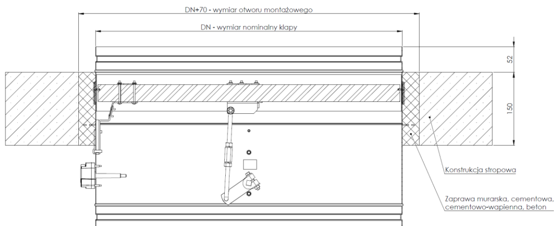
Rys. 3. Sposób zabudowy klap odcinających KTS w konstrukcjach stropowych
