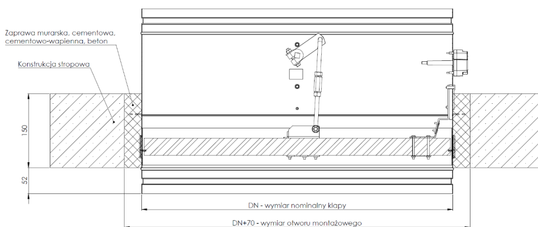
Rys. 4. Sposób zabudowy klap odcinających KTS w konstrukcjach stropowych
